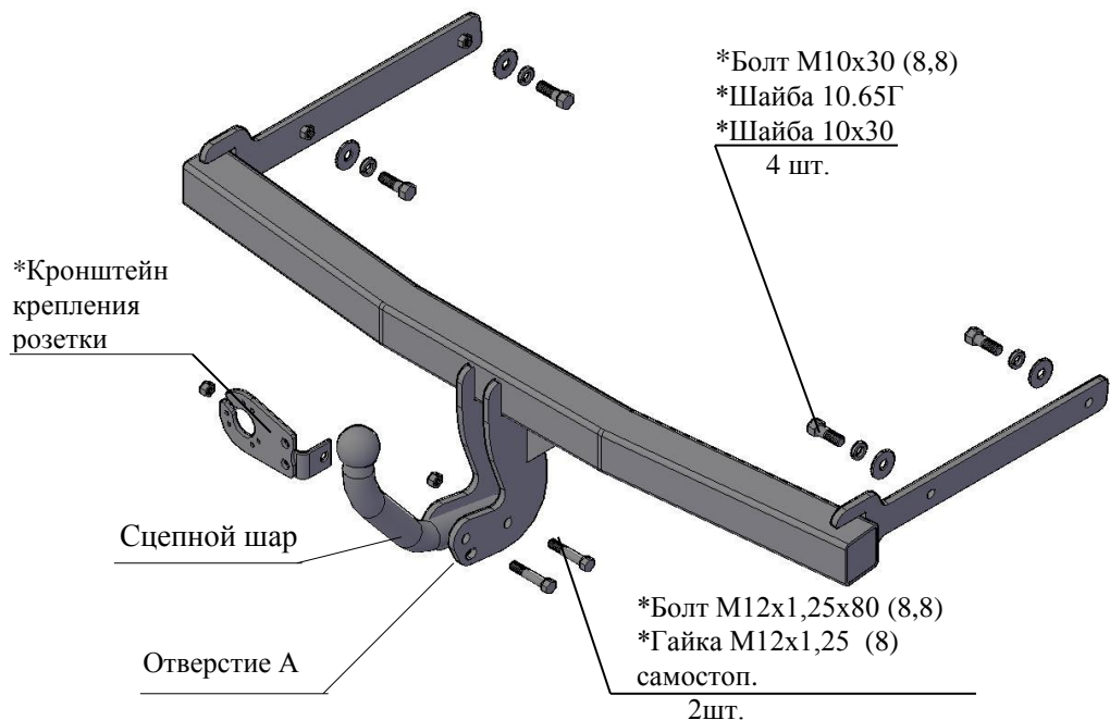
Рис.1 Тягово-сцепное устройство ТСУ 9711.
