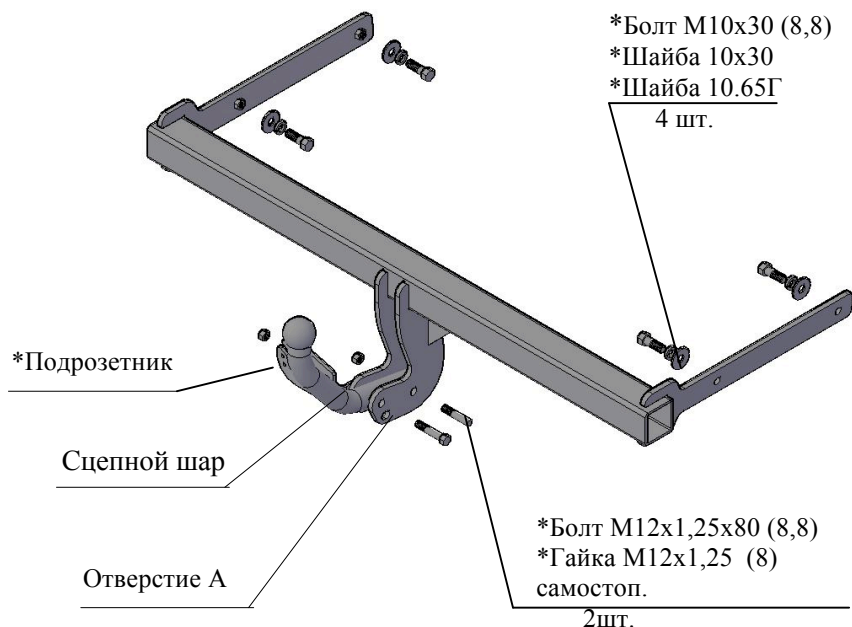
Рис.1 Тягово-сцепное устройство ТСУ 9710.
