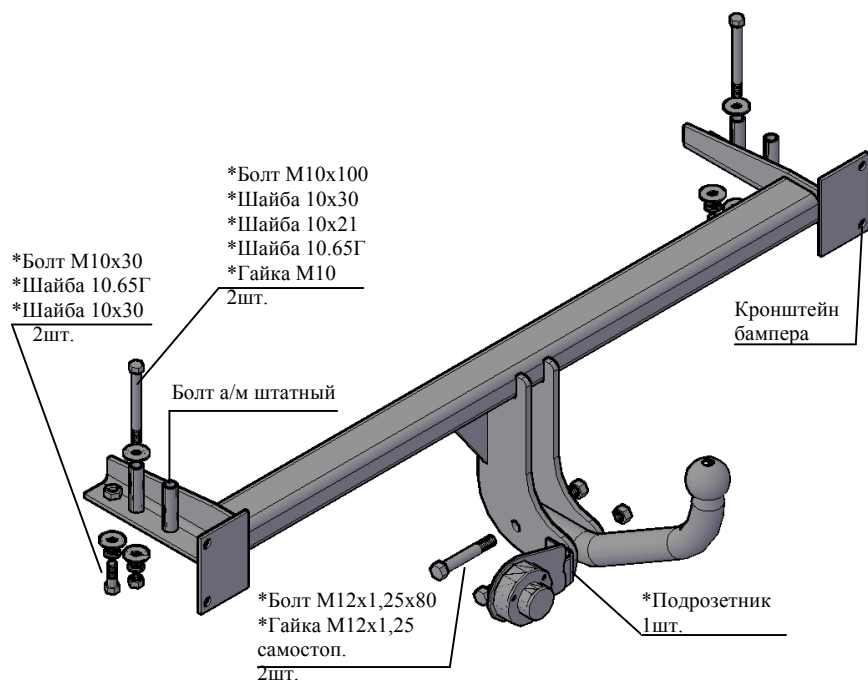
Рис.1 Тягово-сцепное устройство 9420
