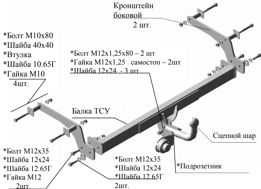
Рис.1 Тягово-сцепное устройство ТСУ 9010 Рено Логан.С.
