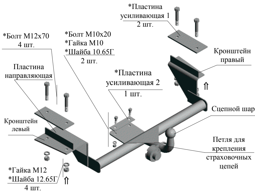
Рис.1 Тягово-сцепное устройство ТСУ 2110
